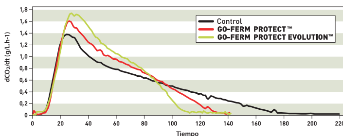
Figure 1: GO-FERM PROTECT EVOLUTION™ impacto en la cinética de fermentación: Lalvin QA23™ (25g/hL) con la adición de protector de levadura (30g/hL) durante la rehidratación en mosto sintético muy clarificado.
